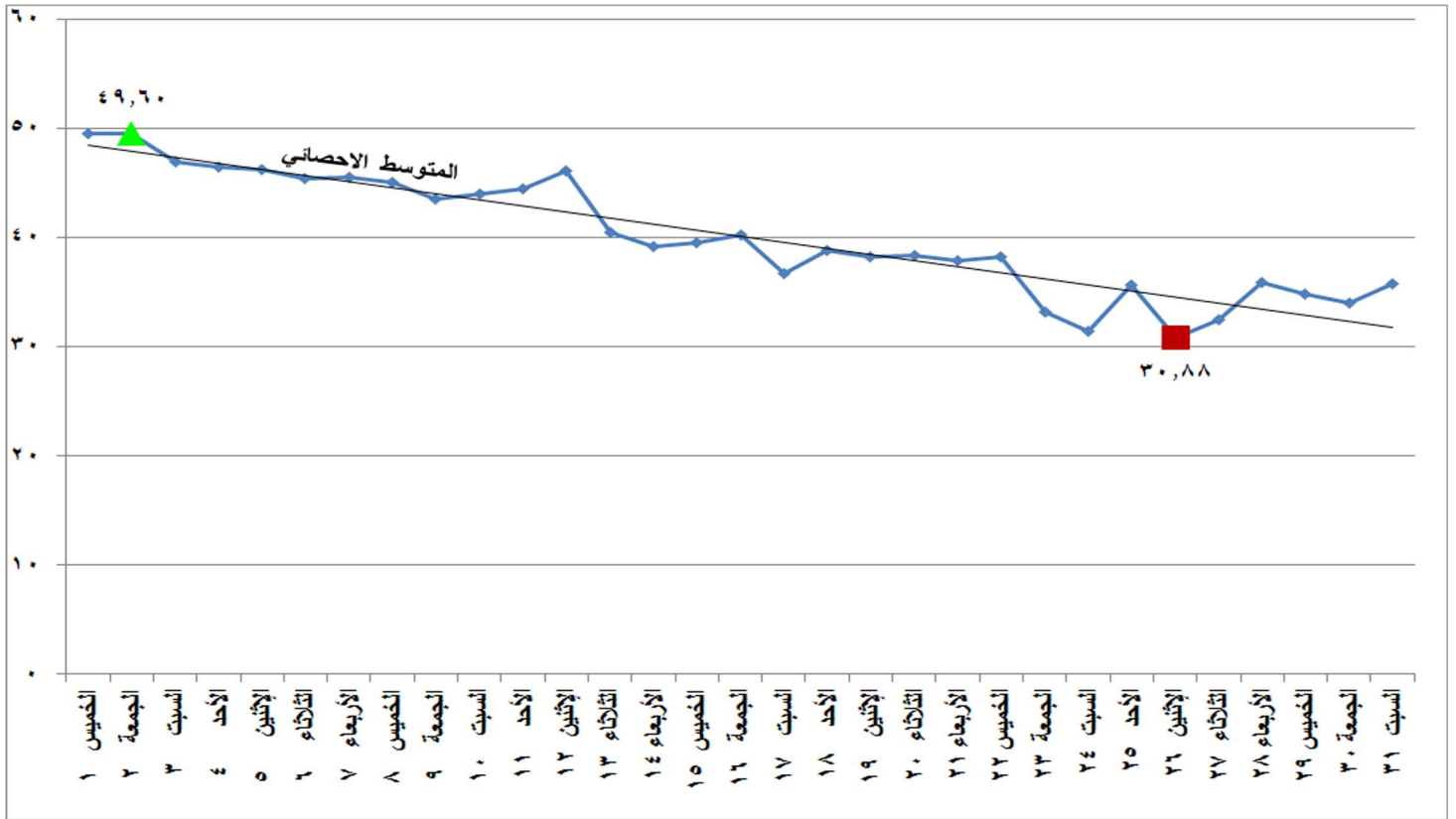
شكل (٢٣) الطاقة الكهربائية المنتجة من المصادر المائية خلال شهر أكتوبر ٢٠٢٠
