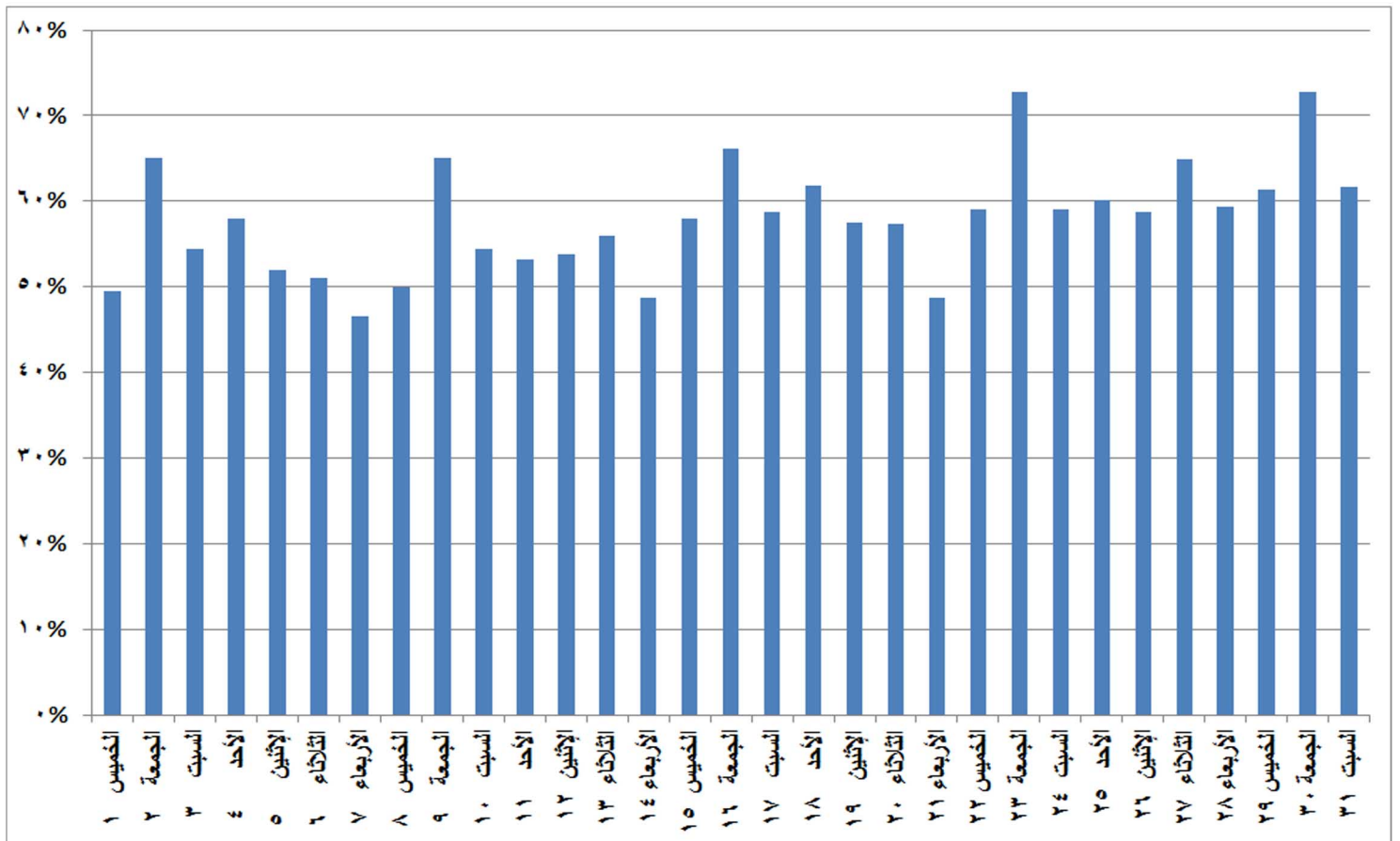
شكل (٢٨) نسب الفائض للحمل الاقصى المسجل يوميا خلال شهر أكتوبر ٢٠٢٠
