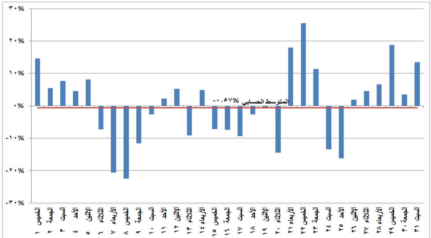
شكل (٢٢) نسب التغير في استخدام المصادر غير الحرارية في إنتاج الطاقة الكهربائية خلال شهر أكتوبر ٢٠٢٠ مقارنة بالشهر المماثل من العام السابق
