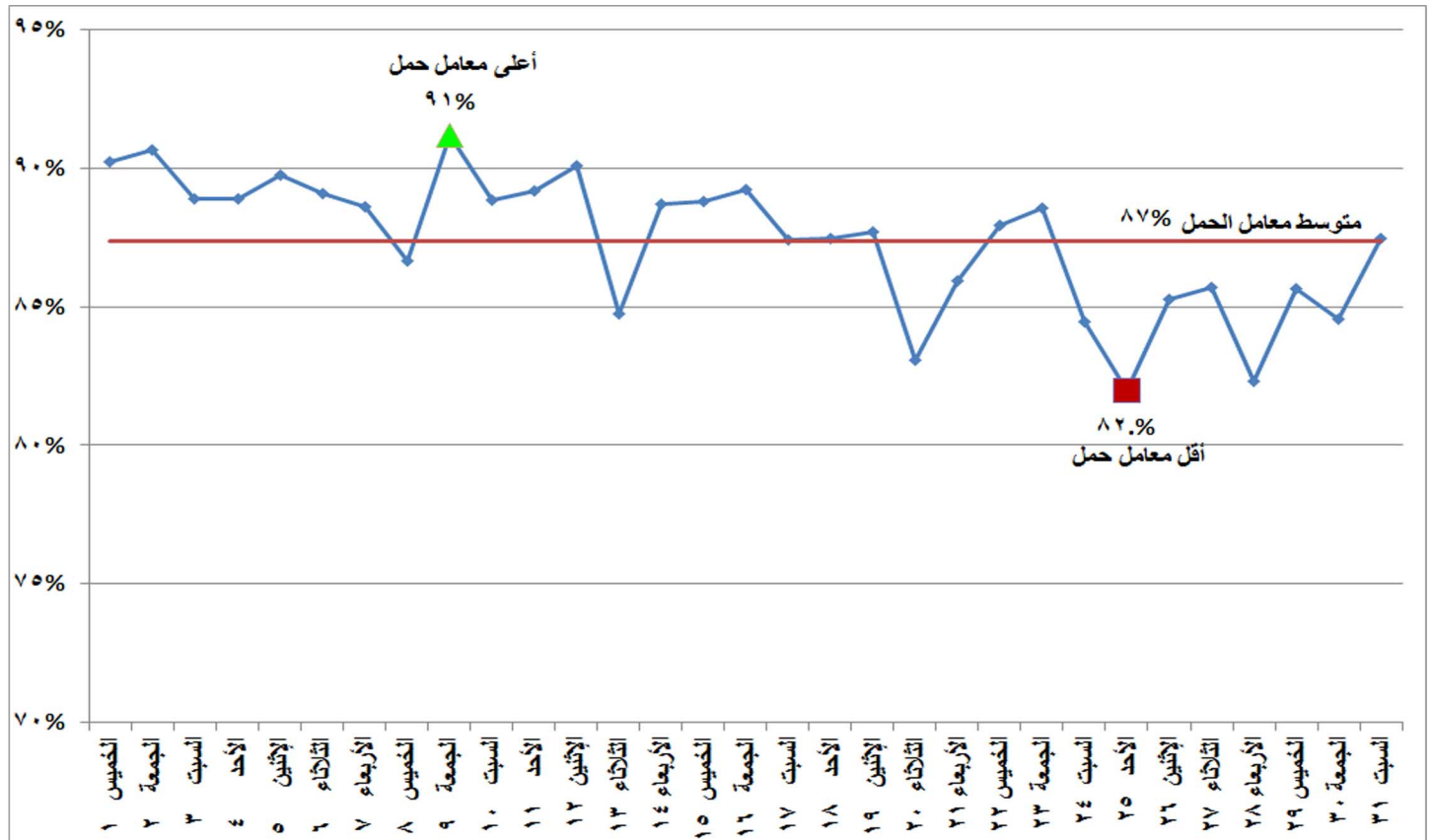
شكل (١٢) إجمالي معامل الحمل لوحدات الانتاج خلال شهر أكتوبر ٢٠٢٠
