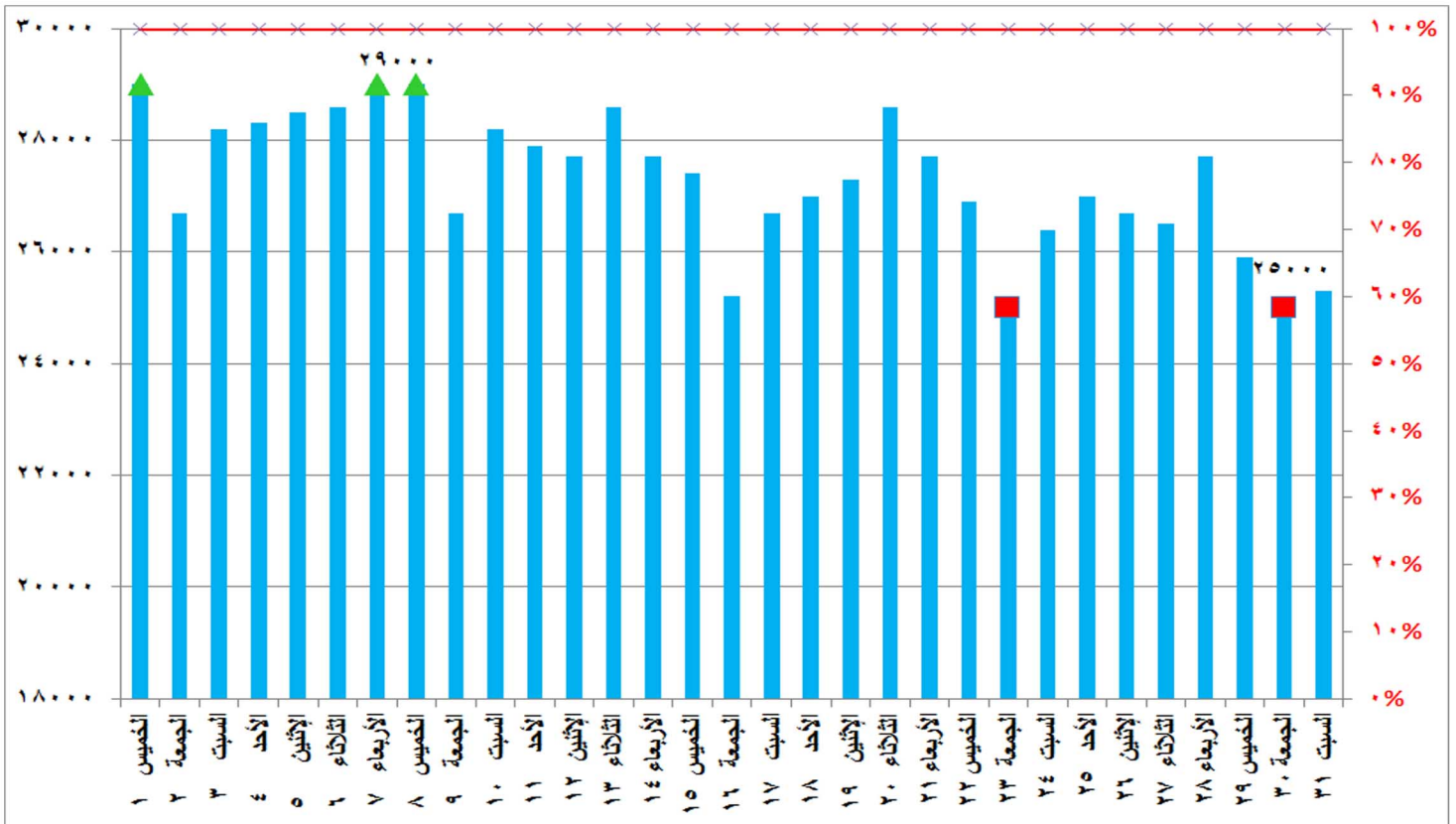
شكل (٥) قدرات الانتاج المتاحة ونسبتها للحمل الأقصى خلال شهر أكتوبر ٢٠٢٠
