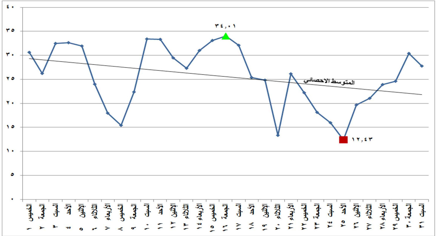
شكل (٢٥) الطاقة الكهربائية المنتجة من الرياح والشمس خلال شهر أكتوبر ٢٠٢٠
