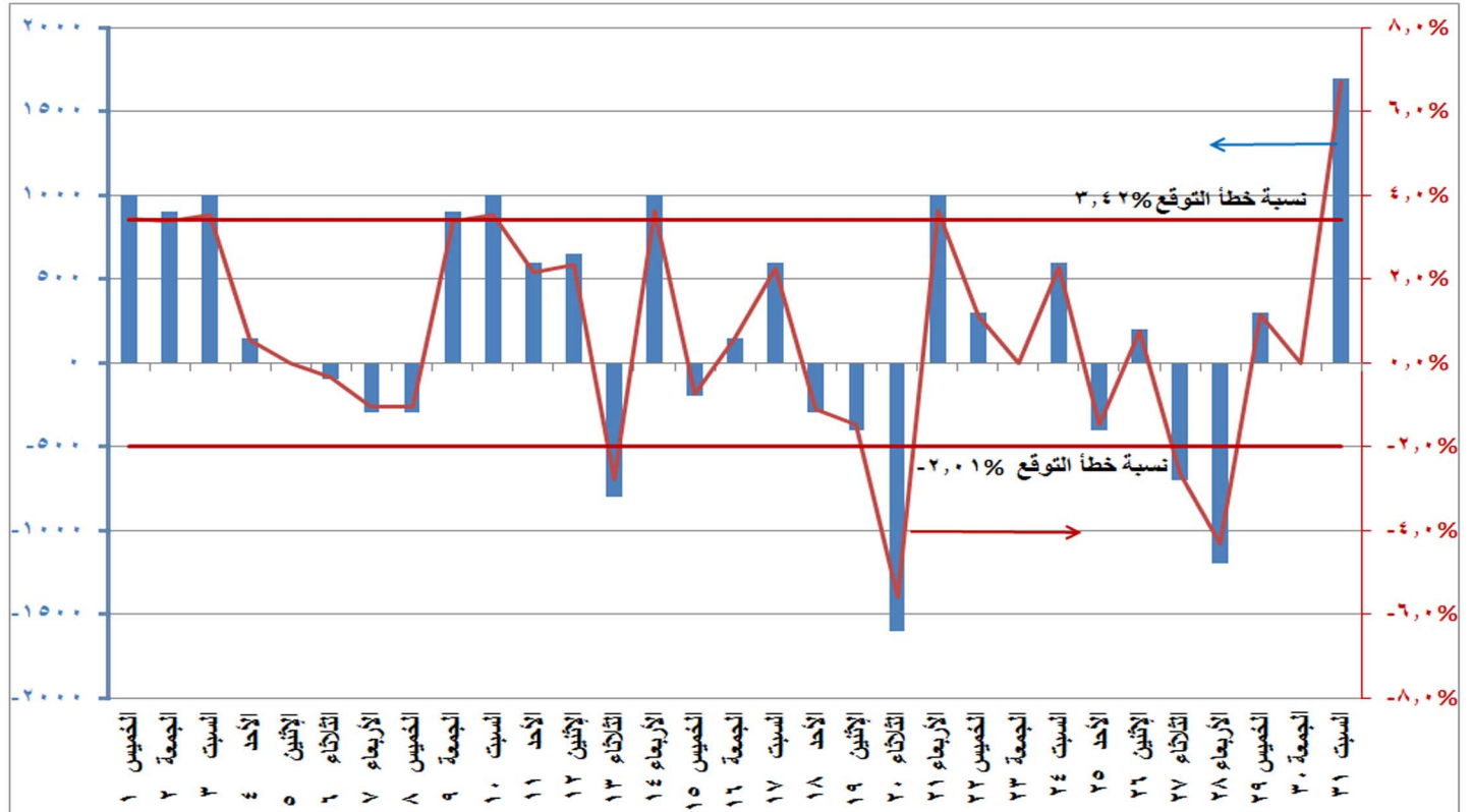
شكل (١٠) الفرق بين الحمل الأقصى المتوقع والمسجل فعليا ونسبة الفرق إلى الحمل المسجل فعليا خلال شهر أكتوبر ٢٠٢٠
