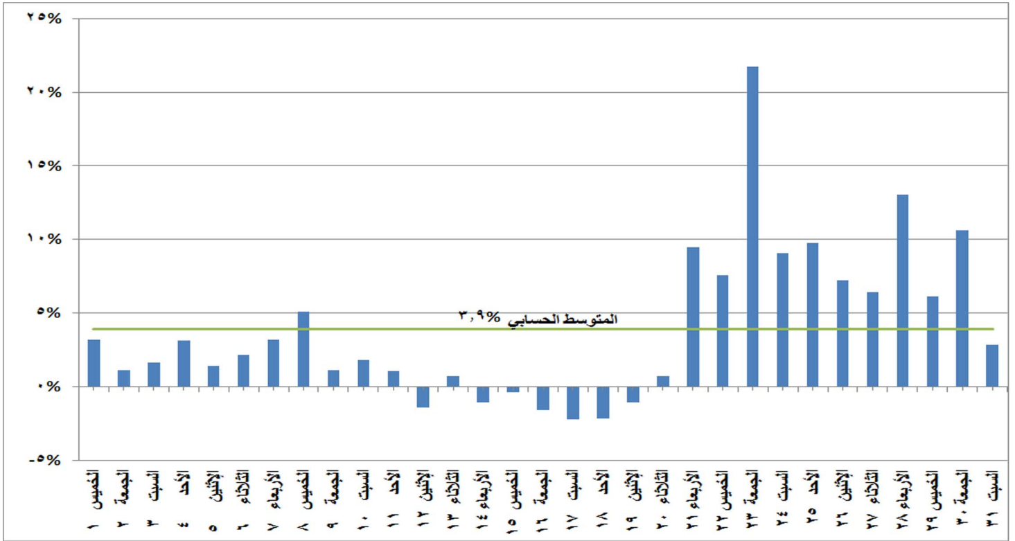
شكل (٩) النسب المئوية للتغير في الحمل الاقصى خلال شهر أكتوبر ٢٠٢٠ مقارنة باليوم المماثل من العام الماضي
