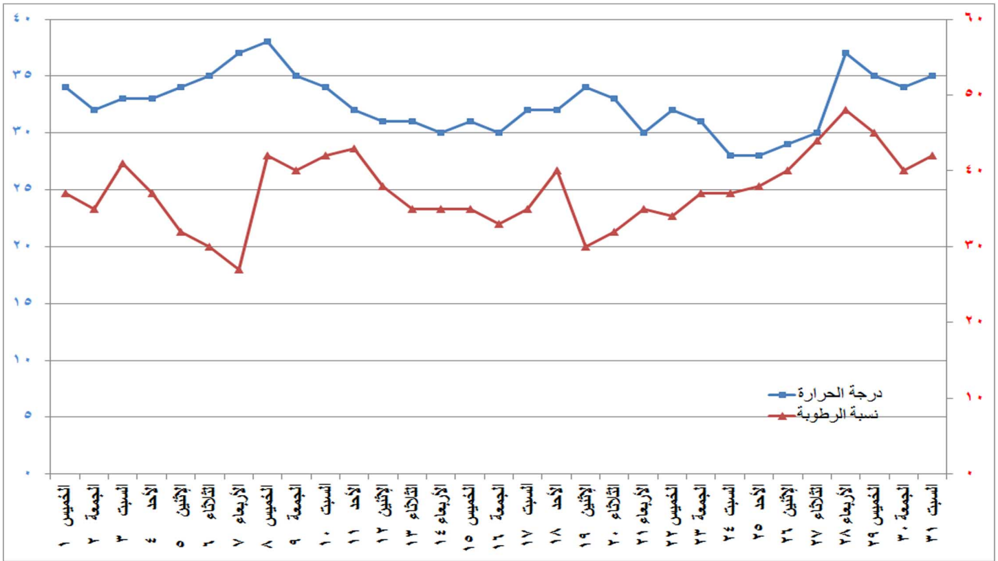
شكل (١١) التغيير في درجة الحرارة والرطوبة النسبية خلال شهر أكتوبر ٢٠٢٠
