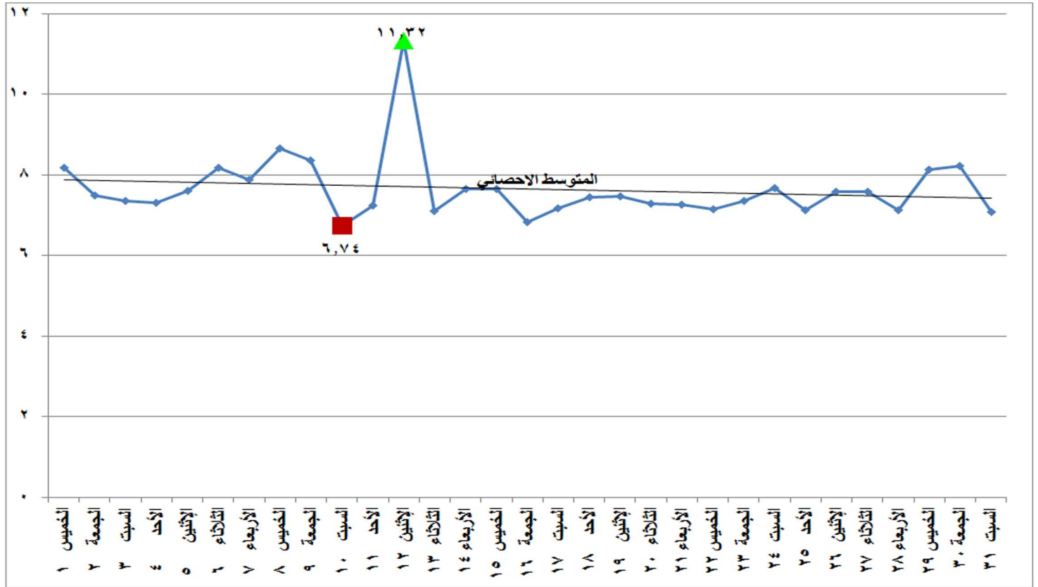
شكل (١٩) الطاقة الكهربائية المنتجة من المازوت خلال شهر أكتوبر ٢٠٢٠
