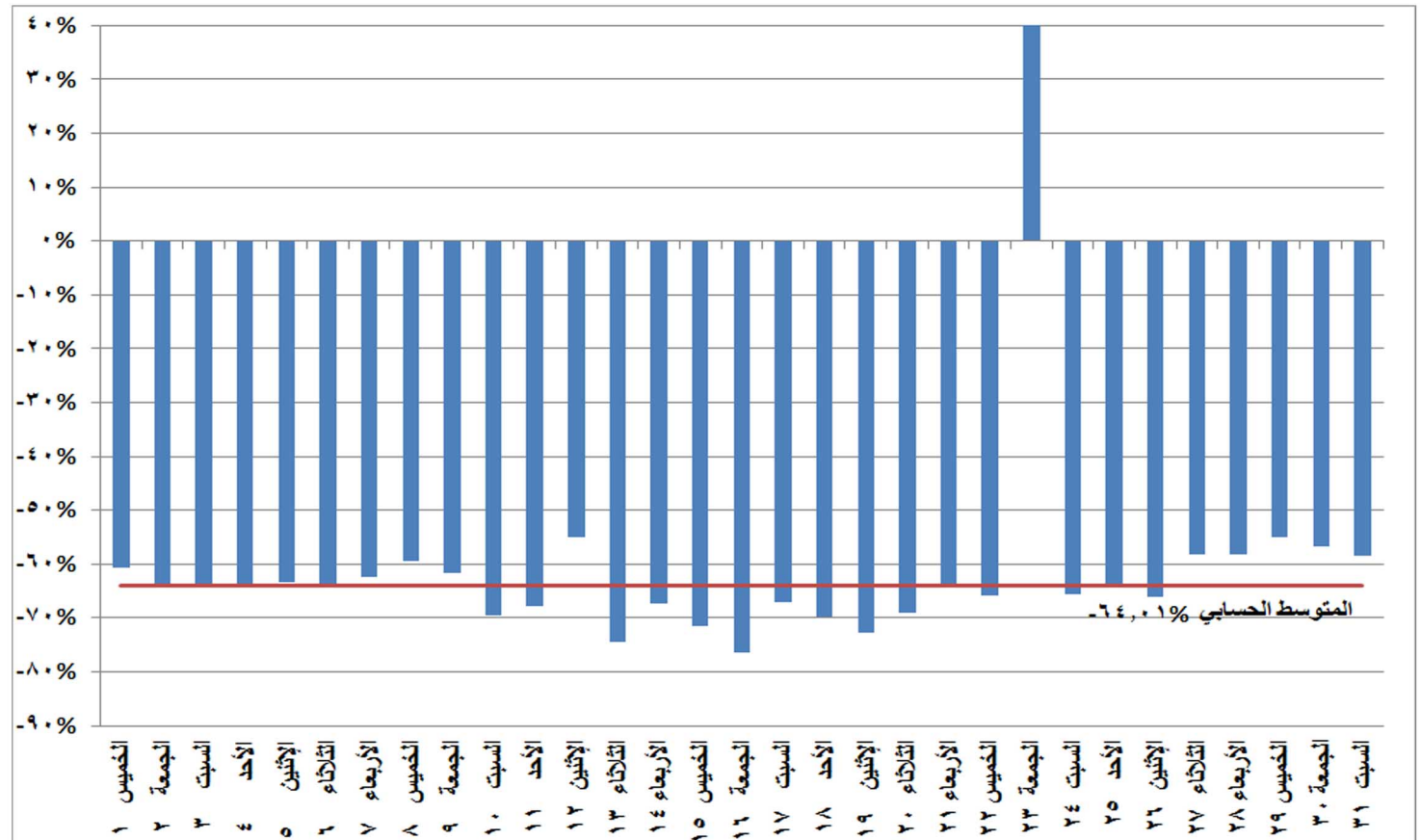
شكل (٢٠) نسب التغير في استخدام المازوت في إنتاج الطاقة الكهربائية خلال شهر أكتوبر ٢٠٢٠ مقارنة بالشهر المماثل من العام السابق
