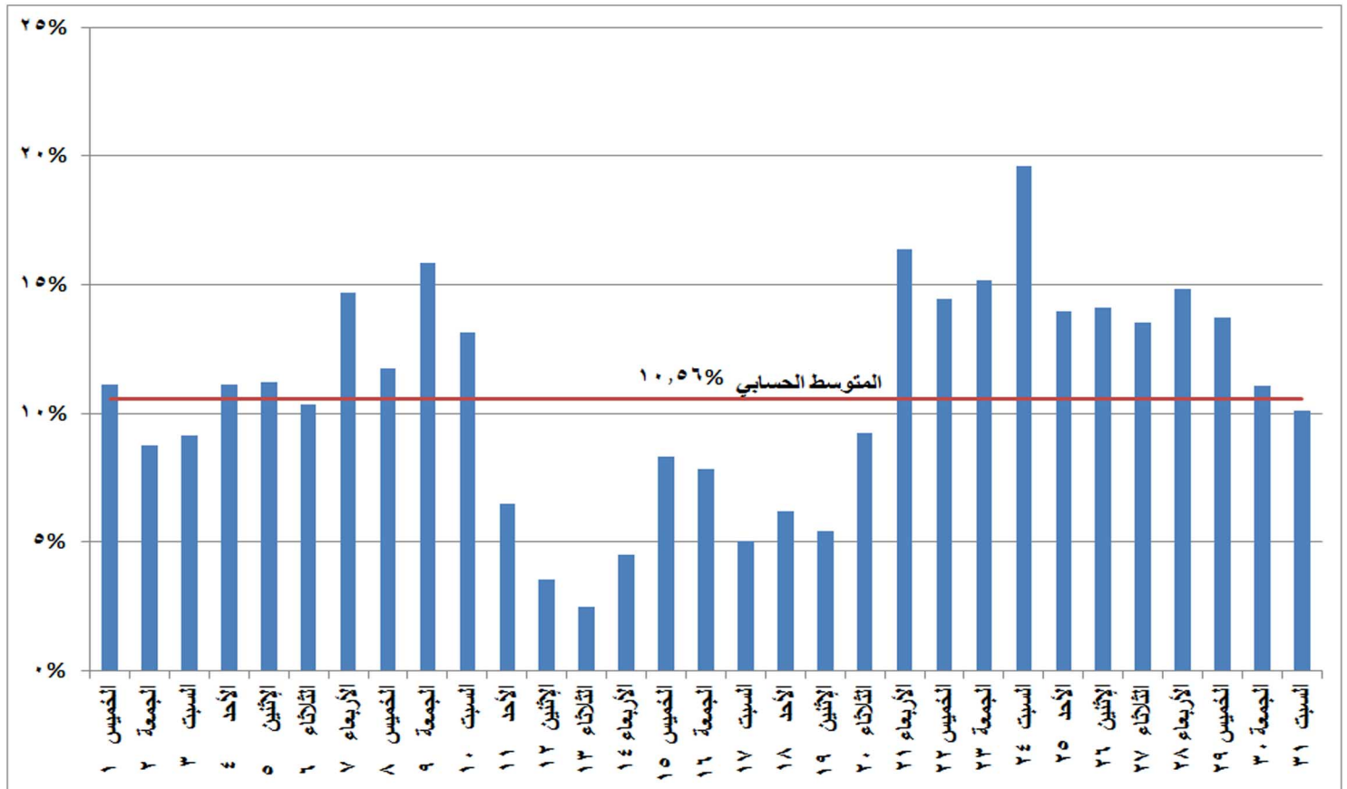
شكل (١٨) نسب التغير في استخدام الغاز الطبيعي في إنتاج الطاقة الكهربائية خلال شهر أكتوبر ٢٠٢٠ مقارنة بالشهر المماثل من العام السابق
