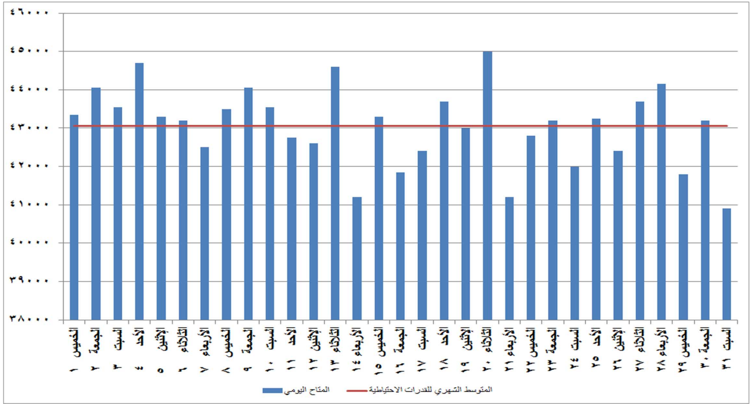
شكل (٢٧) القدرات المتاحة يوميا والمتوسط الشهري للقدرة الاحتياطية خلال شهر أكتوبر ٢٠٢٠
