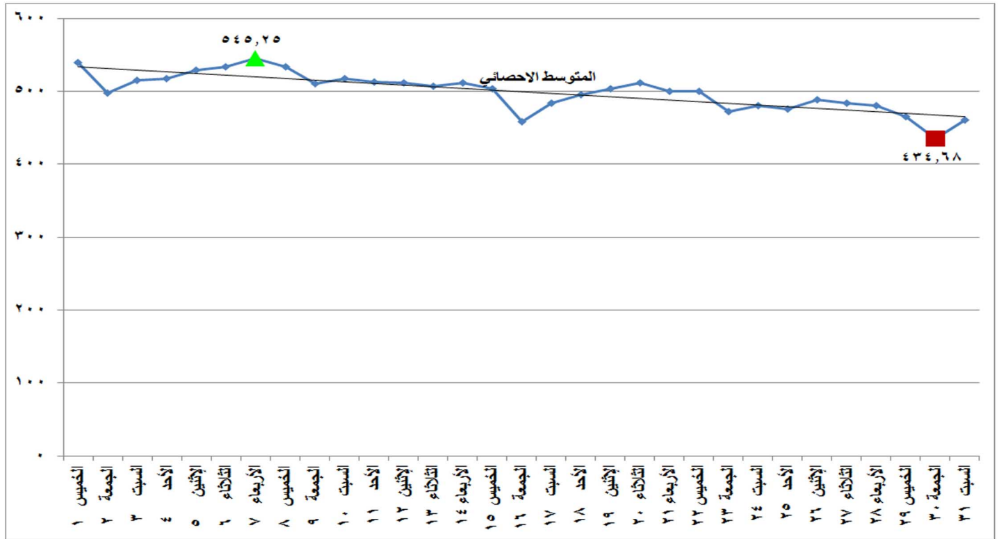
شكل (١٧) الطاقة الكهربائية المنتجة من الغاز الطبيعي خلال شهر أكتوبر ٢٠٢٠
