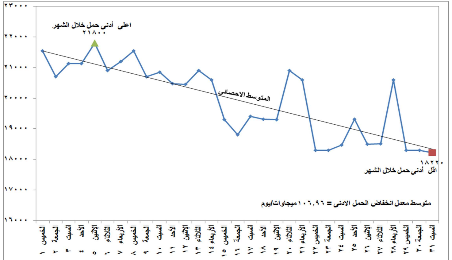
شكل (٢) تطور الحمل الادنى اليومي خلال شهر أكتوبر ٢٠٢٠
